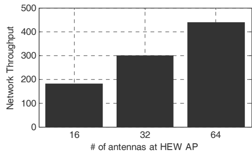
그림 5. 안테나 수에 따른 제안한 JS DR 기법 성능 Fig. 5. Performance of the proposed JS DR (# of antennas at HEW AP)
