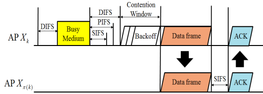
그림 2. IEEE 802.11 매체 접속 제어 방식 Fig. 2. IEEE 802.11 medium access control
