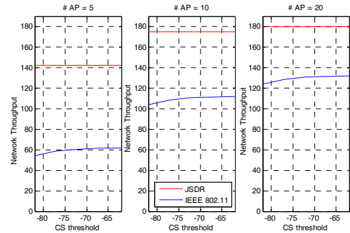
그림 4. 캐리어 센싱 한계값에 따른 제안한 JS DR 성능 Fig. 4. Performance of the proposed JS DR (carrier sensing threshold)
