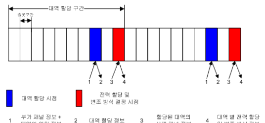
그림 2. 제안한 적응 송신 방식
