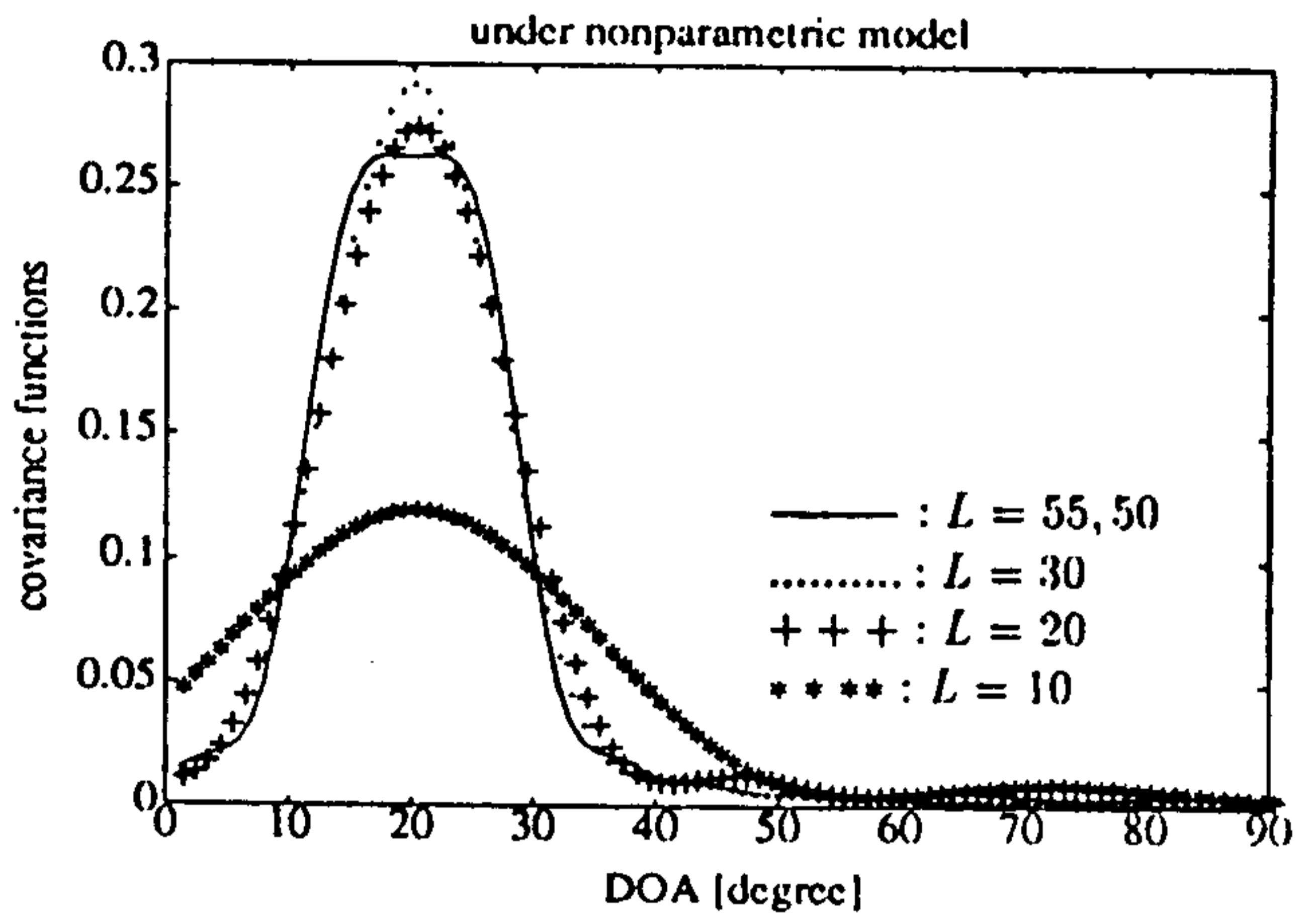
그림 1(나). 배열감지기 수 L 이 55, 50, 30, 20, 10일 때, 그림 1(가)의 퍼진신호원의 공분산 함수들.
