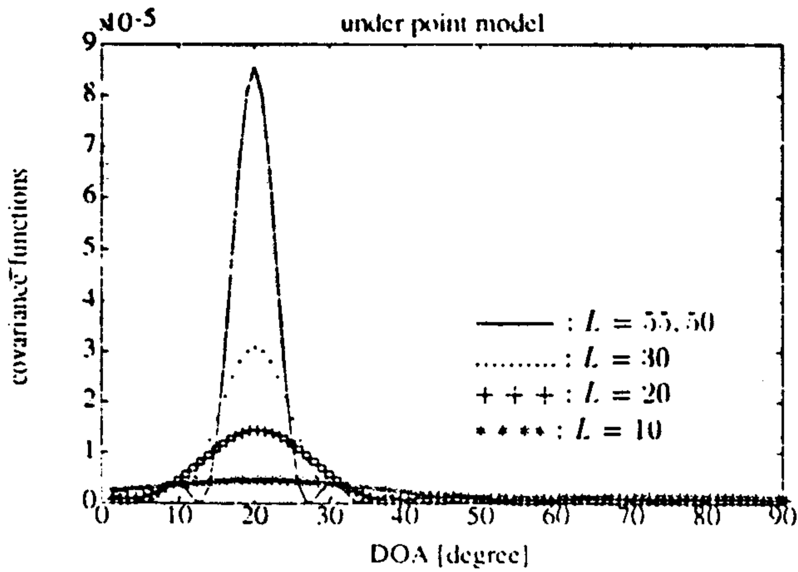
그림 2. 배열감지기 수 L 이 55, 50, 30, 20, 10일때, 점신호원 밀도 S(\theta, t) = \delta(\theta - \frac{\pi}{9}) 의 공분산 함수들
